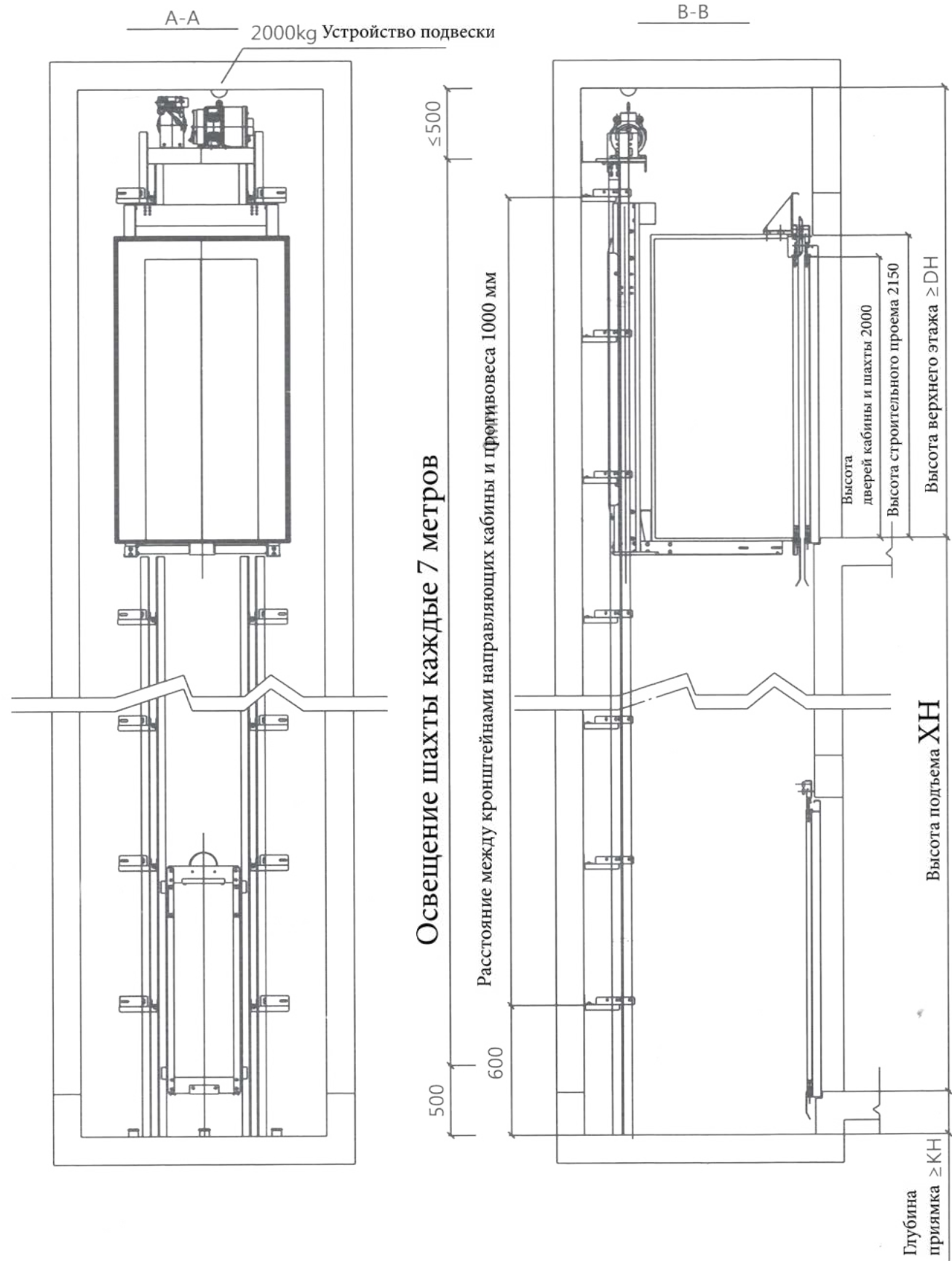
План шахты
